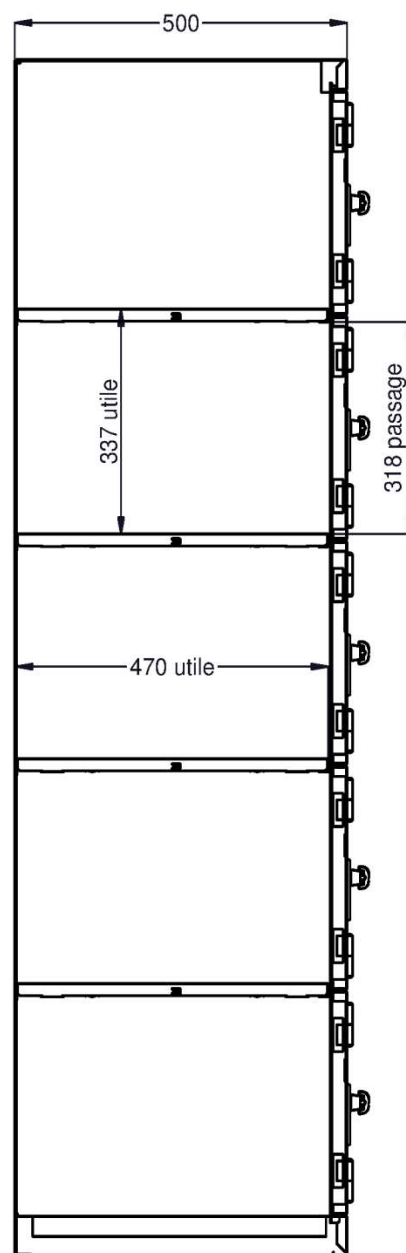
COUPE DE COTE
